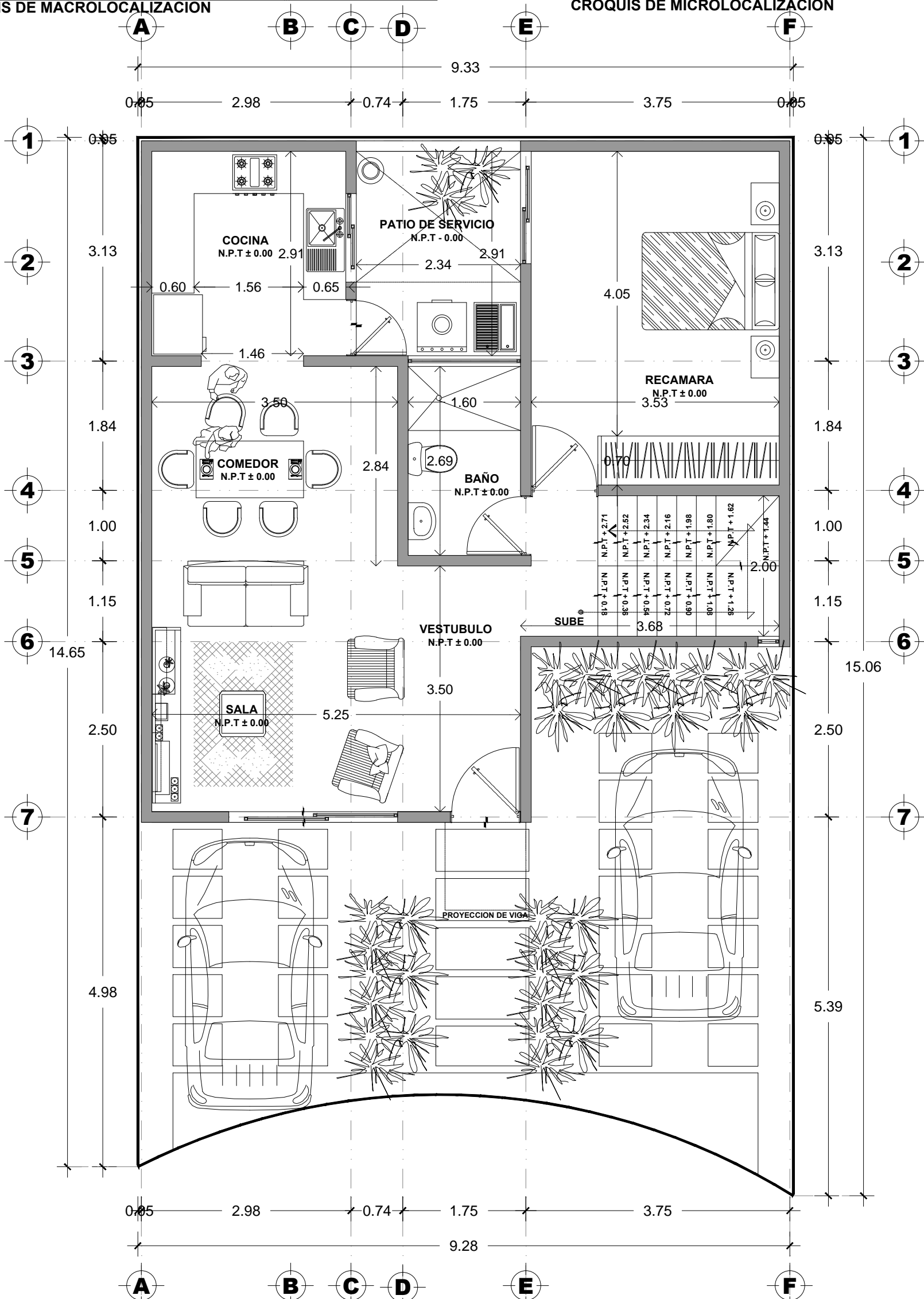
PLANTA ARQUITECTONICA BAJA LOTE 2, FRACCIONAMIENTO RESIDENCIAL "LA FLORESTA"
