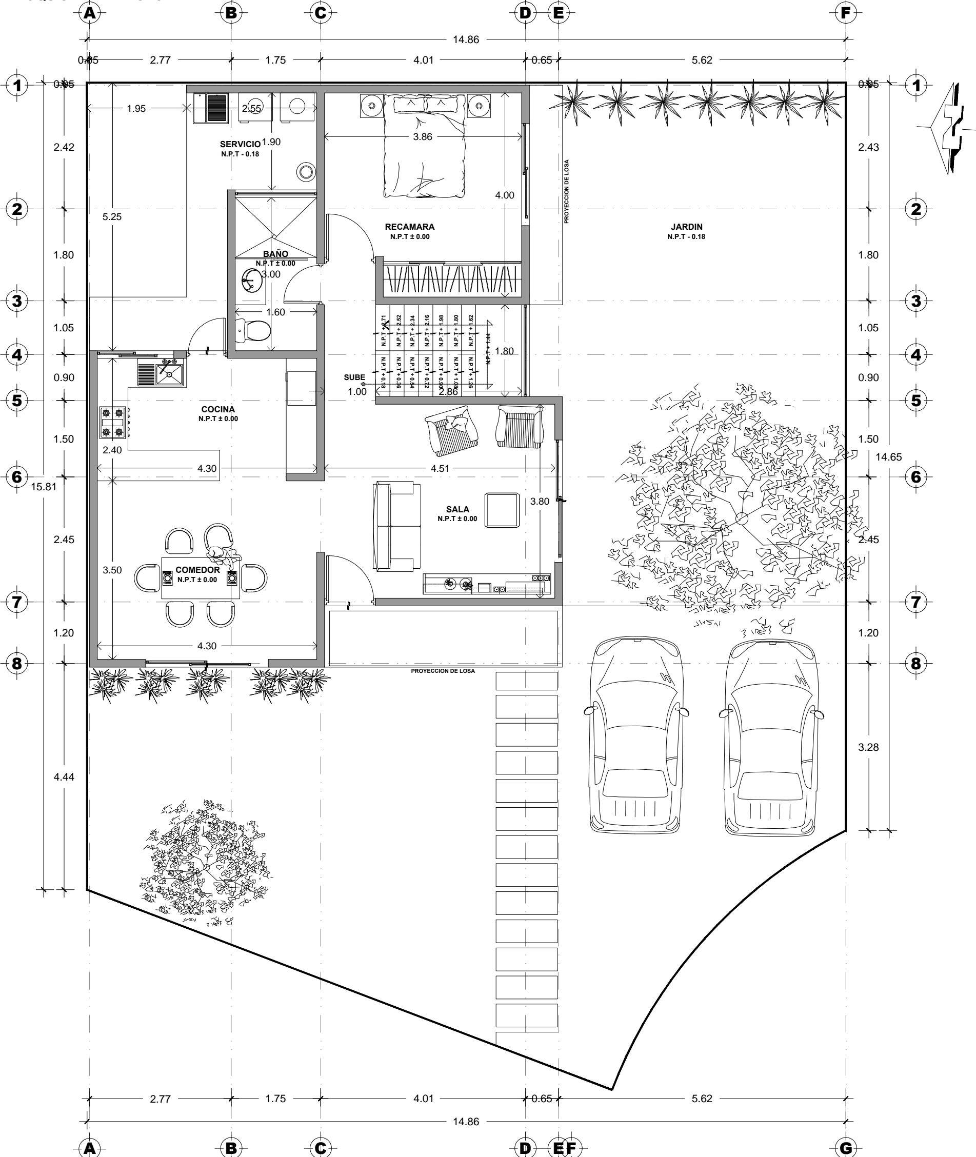
PLANTA ARQUITECTONICA BAJA LOTE 3, FRACCIONAMIENTO RESIDENCIAL "LA FLORESTA"
