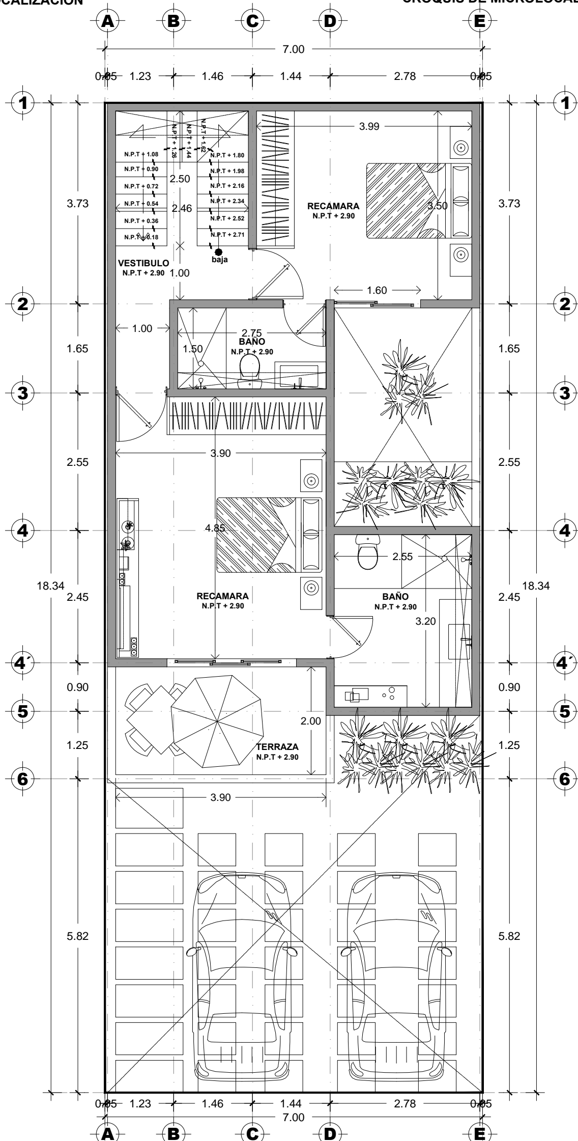
PLANTA ARQUITECTONICA ALTA LOTE 6-11, FRACCIONAMIENTO RESIDENCIAL "LA FLORESTA"
