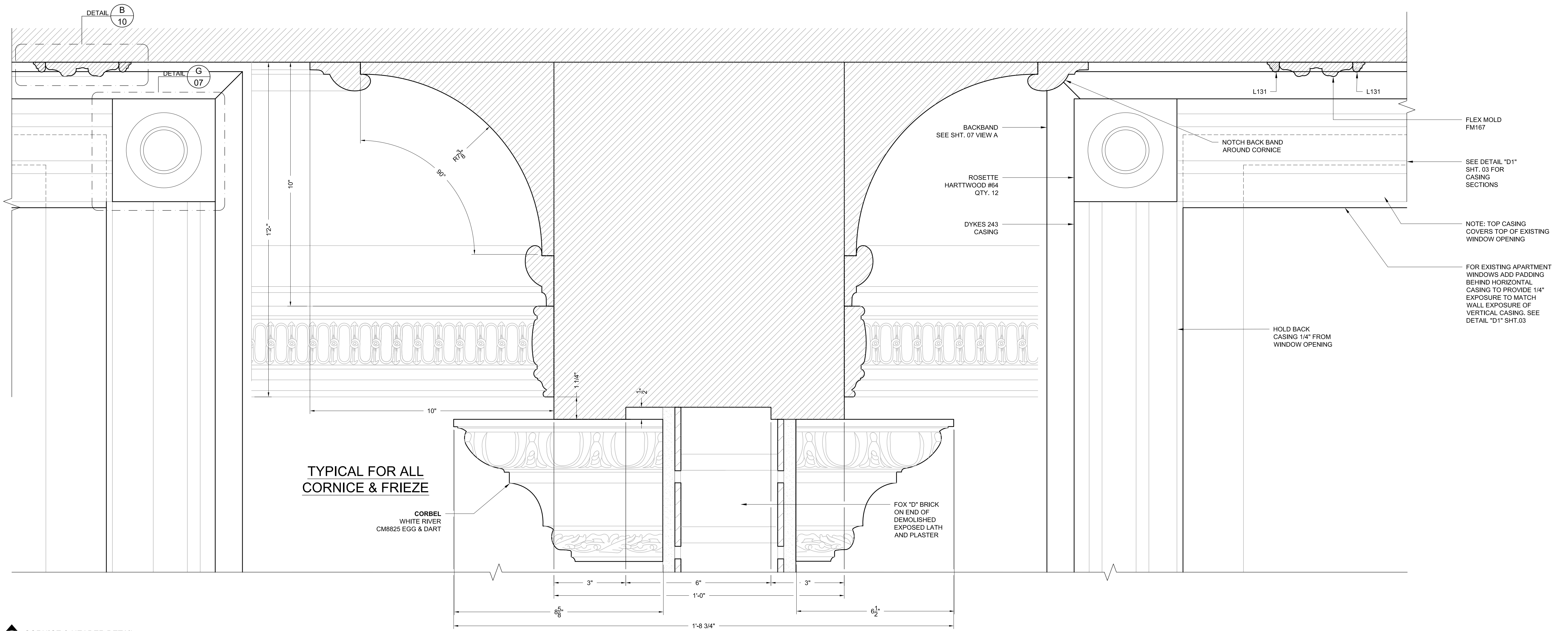
A1 CORNICE & HEADER DETAIL SCALE: 6\"=1'-0\"
