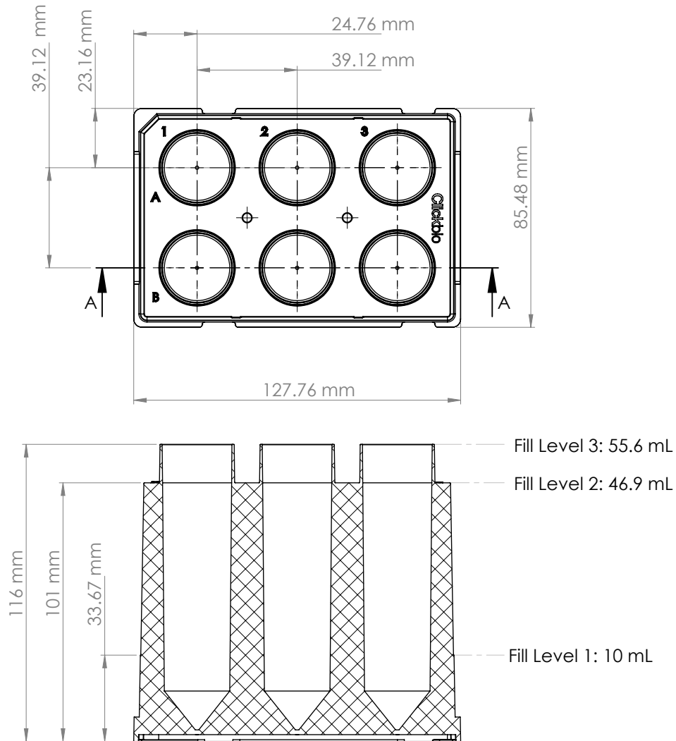
SECTION A-A
