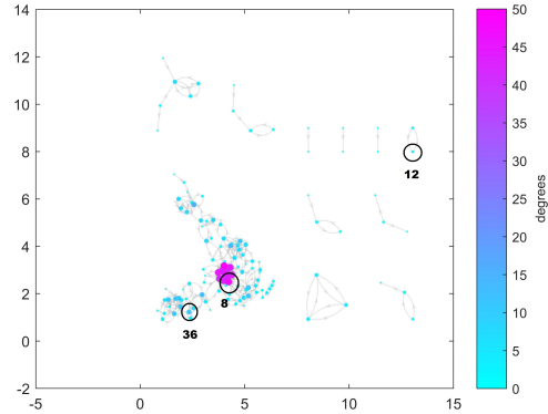
(b) True
