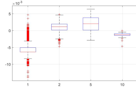
(d) \beta
