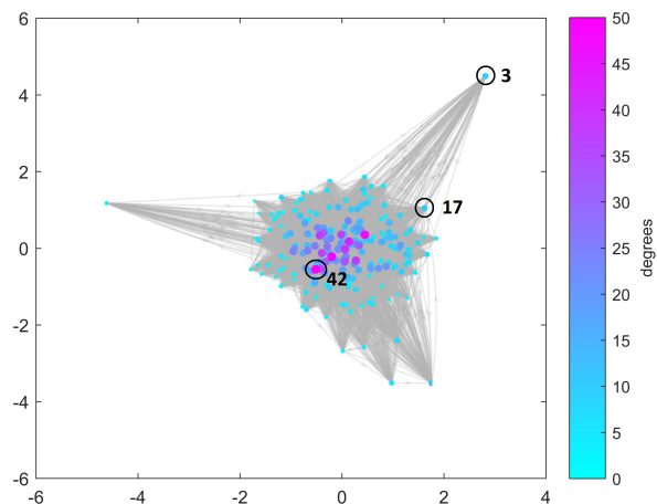
(b) True
