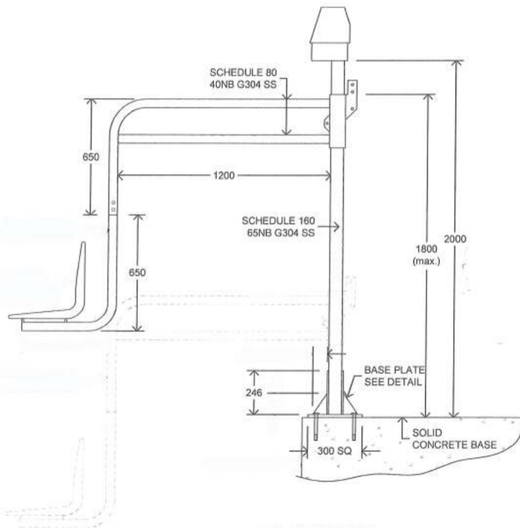
ELEVATION 1:20
