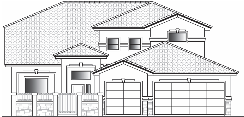
ELEVATION A
