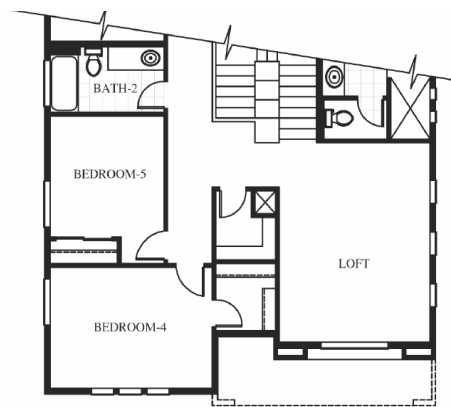
OPTIONAL BEDROOM 5
