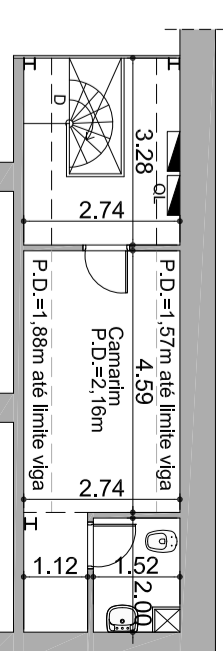
PLANTA - ESTAÇÃO SÃO PAULO CAMARIM escala gráfica 0 1 2 3 4 5
