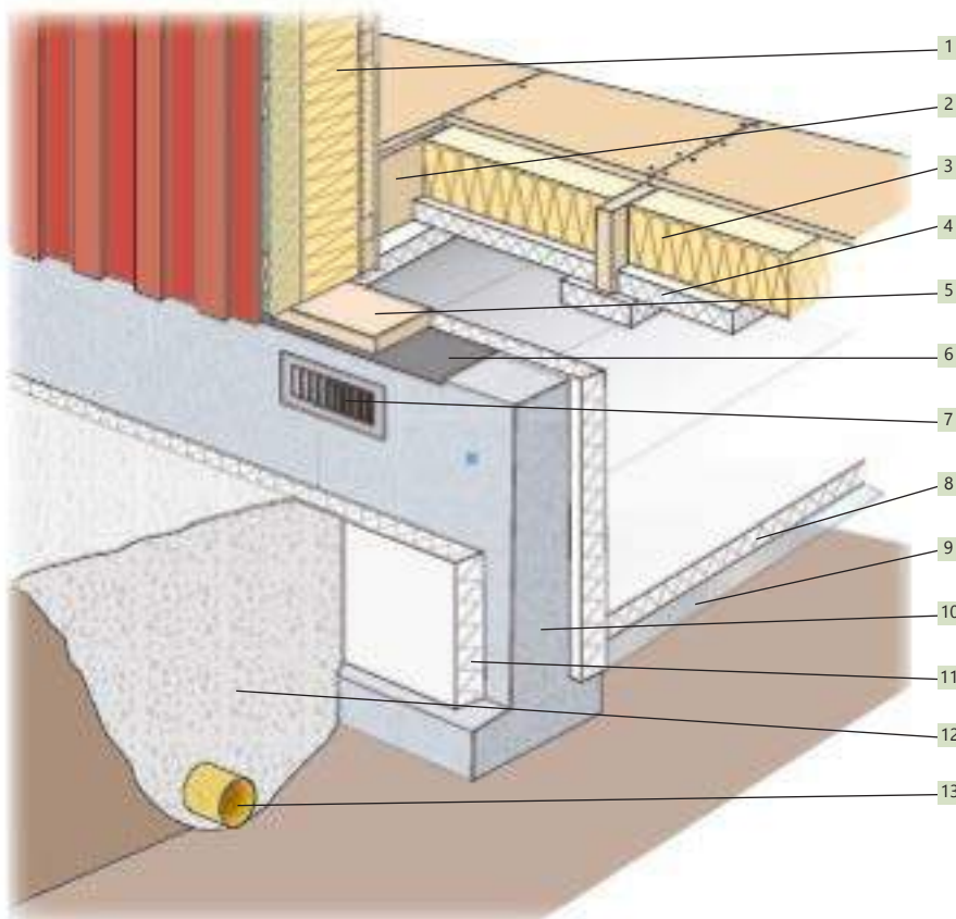
Exempel på uteluftsventilerad krypgrund. U-värde på 0,12 W/(m 2 •K)
