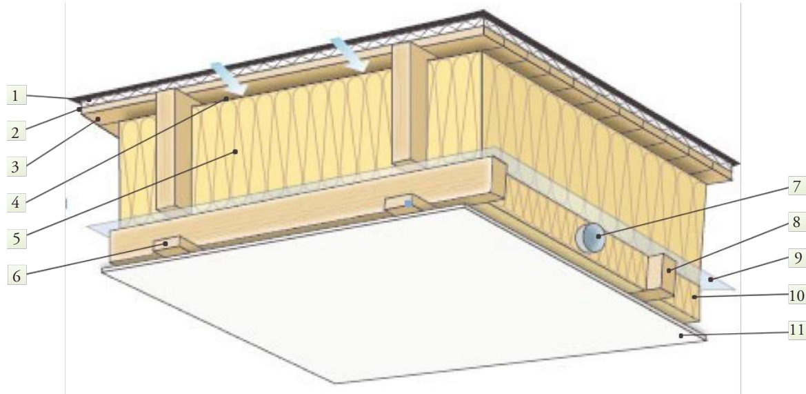
Exempel på låglutande yttertak med utvändig värmeisolering och rördragningar innanför ångspärren. U-värde: 0,09 W/(m 2 .K)
