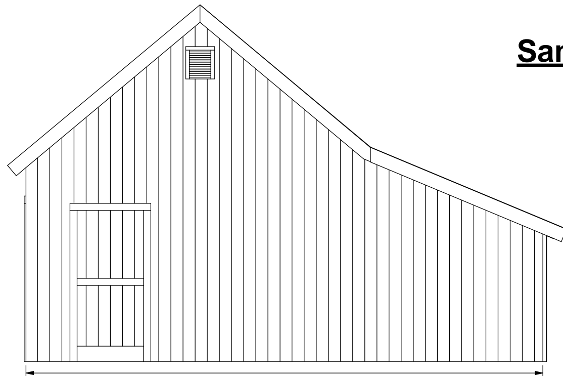
Right Elevation
