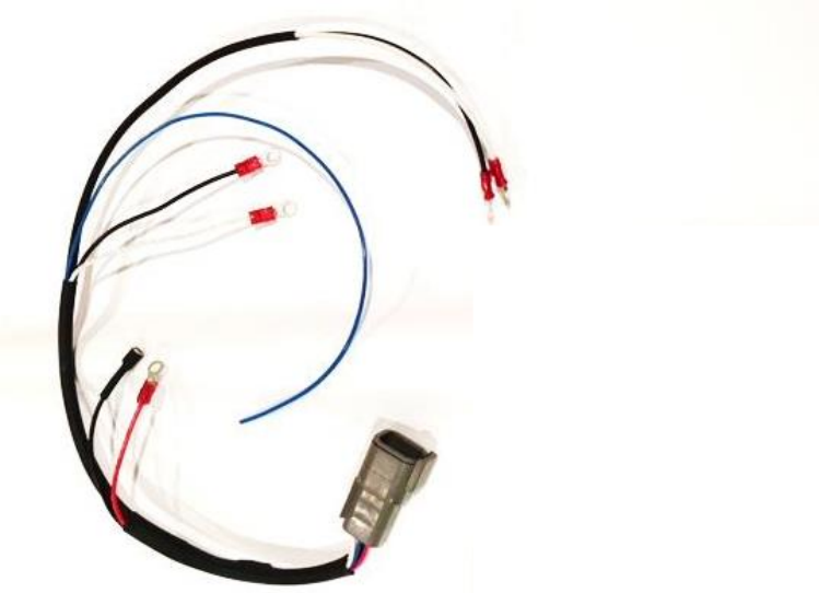
Figure A5 – G3 Dash Harness
