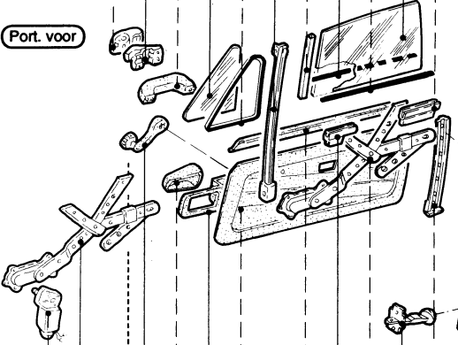
ruitbediening elektr.
