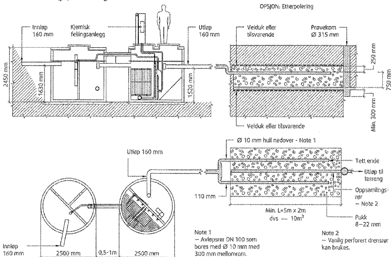
Fig. 1 Plan og snitt av rensesanlegget
