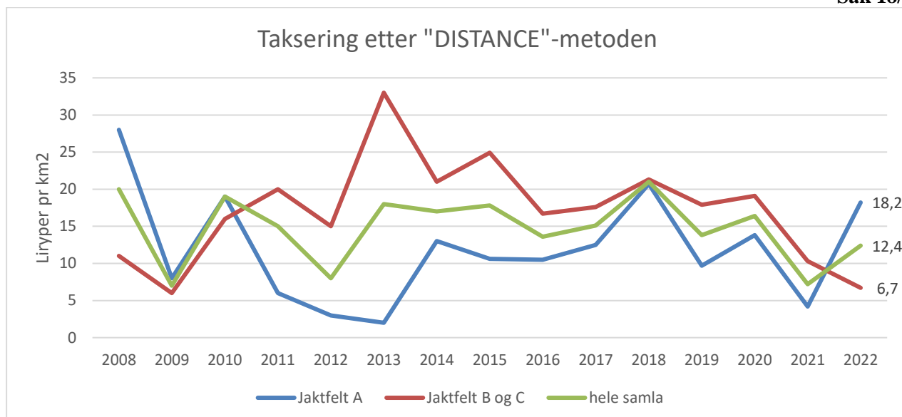
Figur 4. Takstresultat fordelt på jaktfelt og samla for hele statsallmenningen. Jaktfelt A er i sør og jaktfelt B/ midt og nord. Begge områder viste en nedgang i 2021. I år ser vi et bedre takstresultat i den sørre del av statsallmenningen, et område som tidligere har hatt lavere tetthet enn områdene lenger nord.
