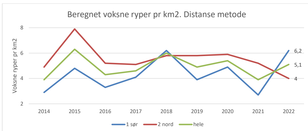
Figur 5. Voksne ryper pr. km 2 fordelt på jaktfelt og samla for hele statsallmenningen. Blå linje viser resultatene for jaktfelt A (sør), rød linje viser resultater for jaktfelt B og C, og grønn linje viser samla verdier. Totalt har beregnet voksne ryper pr km 2 (fig.5) hatt en liten økning fra i fjor, denne økningen skyldes en økning i sør(A). I jaktfelt B og C registrerer vi et svært lavt nivå også av voksne ryper.
