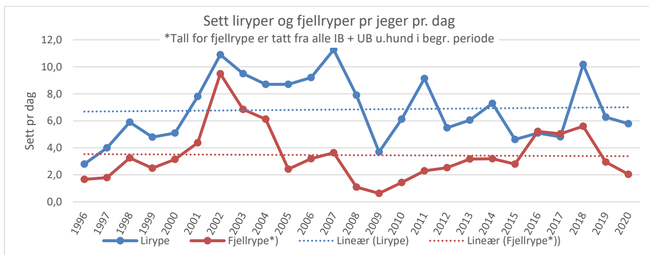
Figur 7. Sett rype pr. jegerdag. Det har vært en nedgang i sette ryper fra 2018. For 2021 har vi ingen data vi kan sammenligne med (siden rypejakta ble avlyst).
