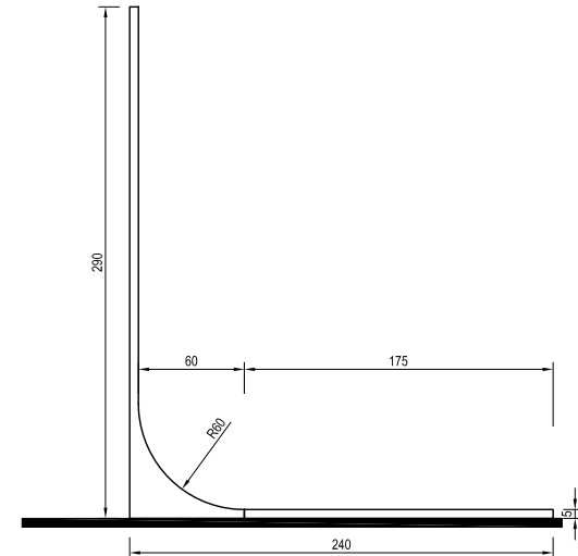
3 SIDE ELEVATION Scale: 1:30
