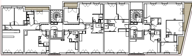
Plan R+2
