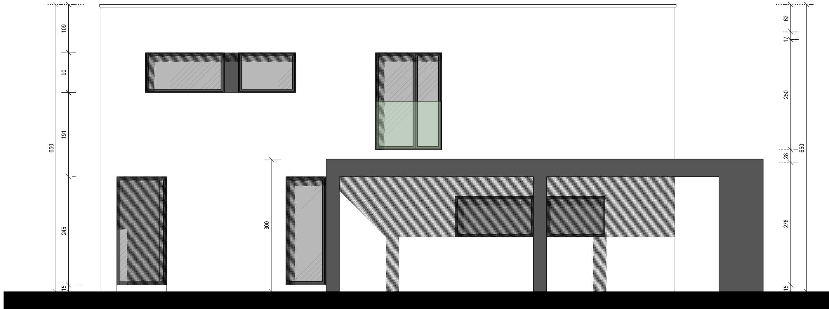
ZIJGEVEL RECHTS - 1/50
