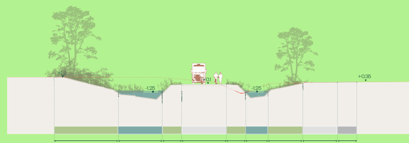
Het voorgestelde profiel van de Euvelgunnerweg en de Hunze.
