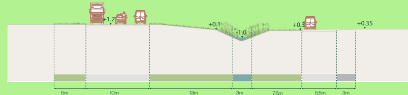
Het oude profiel van de Euvelgunnerweg en de Hunze.
