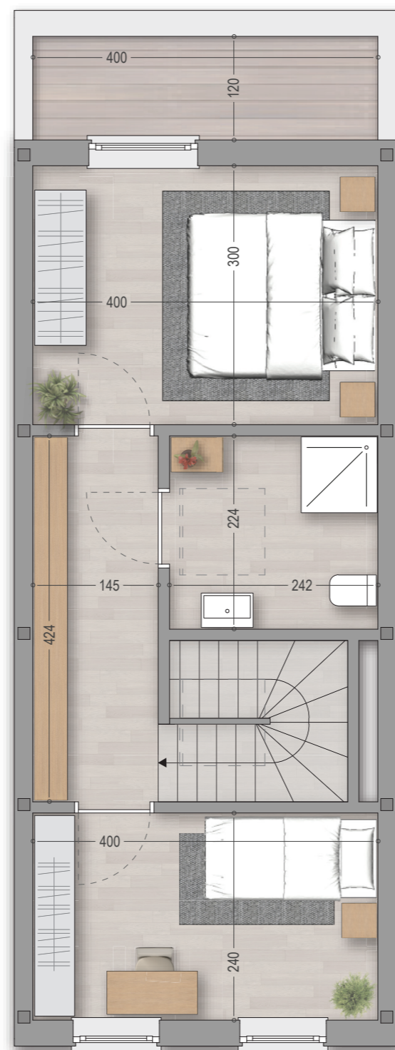
eerste verdieping
