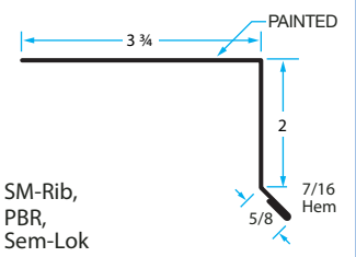
EF-3 Eave Flashing
