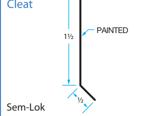
CL-1 Cleat
