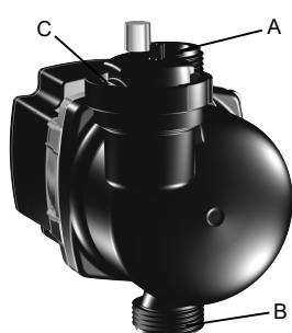
CIAO2 composite, inline, air outlet
