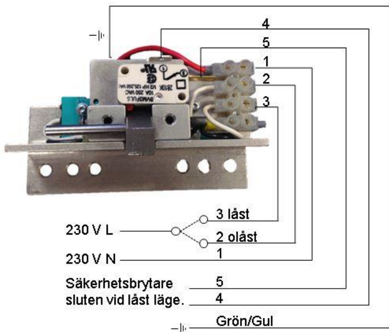
Kopplingsanvisning.
