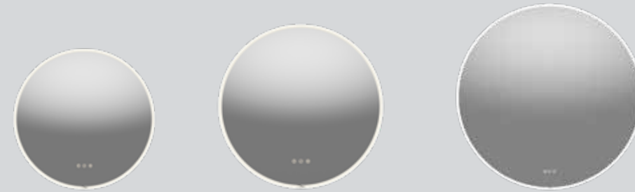
Ø: 60 cm D: 25 mm ut fra vegg Bredde lysfelt: 15 mm Ø: 80 cm D: 25 mm ut fra vegg Bredde lysfelt: 15 mm Ø: 100 cm D: 25 mm ut fra vegg Bredde lysfelt: 15 mm LED/IP44/REG. FARGETEMPERATUR 3000K-6500K 60 CM/16 W/1755 L 80 CM/22 W/2457 L 100 CM/28 W/3121 L
